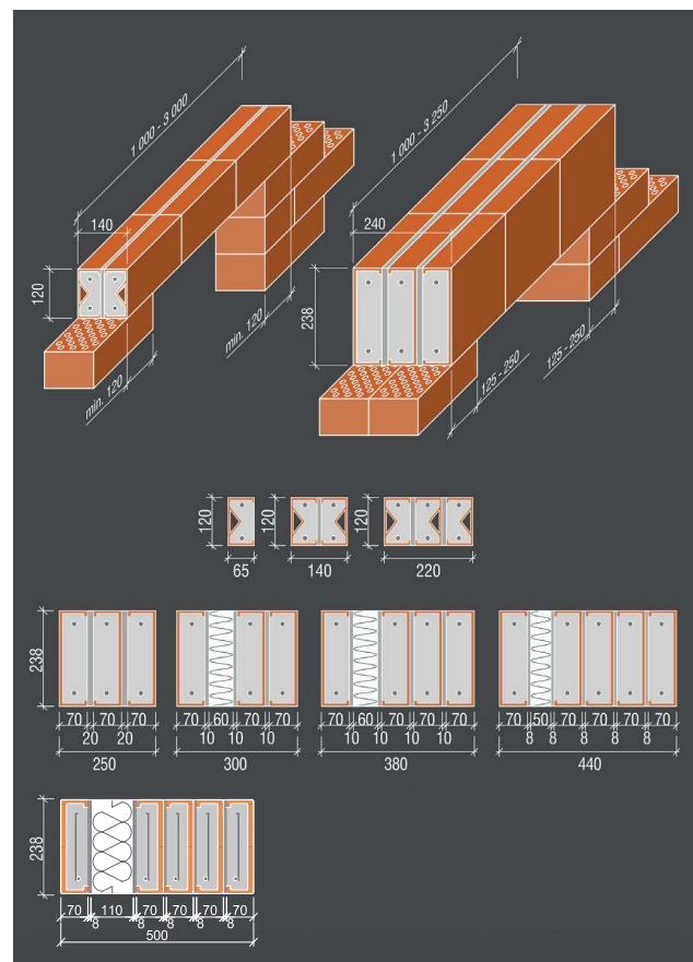
Ukážka použitia keramického prekladu pri preklopení otvoru v rôznej hrúbke muriva
