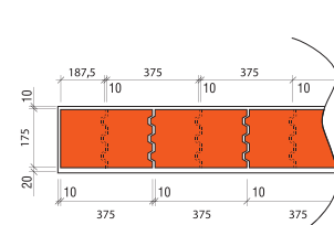
TD 175 PD AKUSTIK
