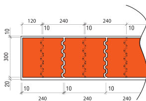
TD 300 PD AKUSTIK
