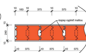
TD 240 PD AKUSTIK ZK
